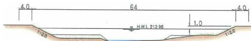
河川整備計画断面図 (吉野川合流点から上流0.3km)
