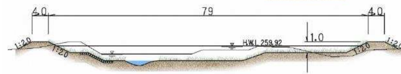
河川整備計画断面図（国道13号から上流0.1km）
