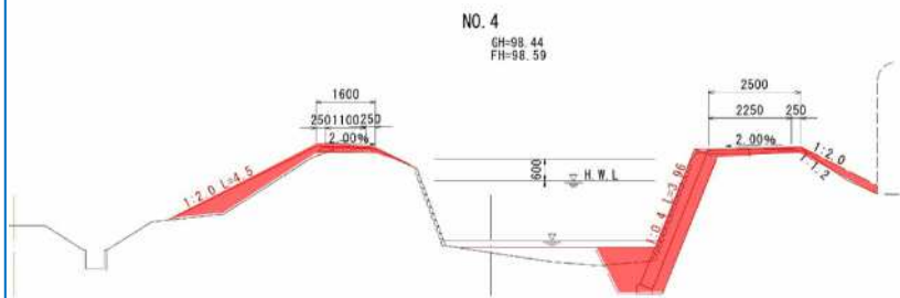
計画断面図
