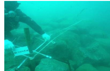
潜水土による目視点検
