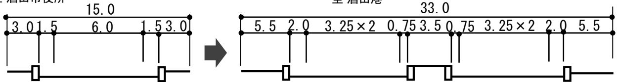
断面図
