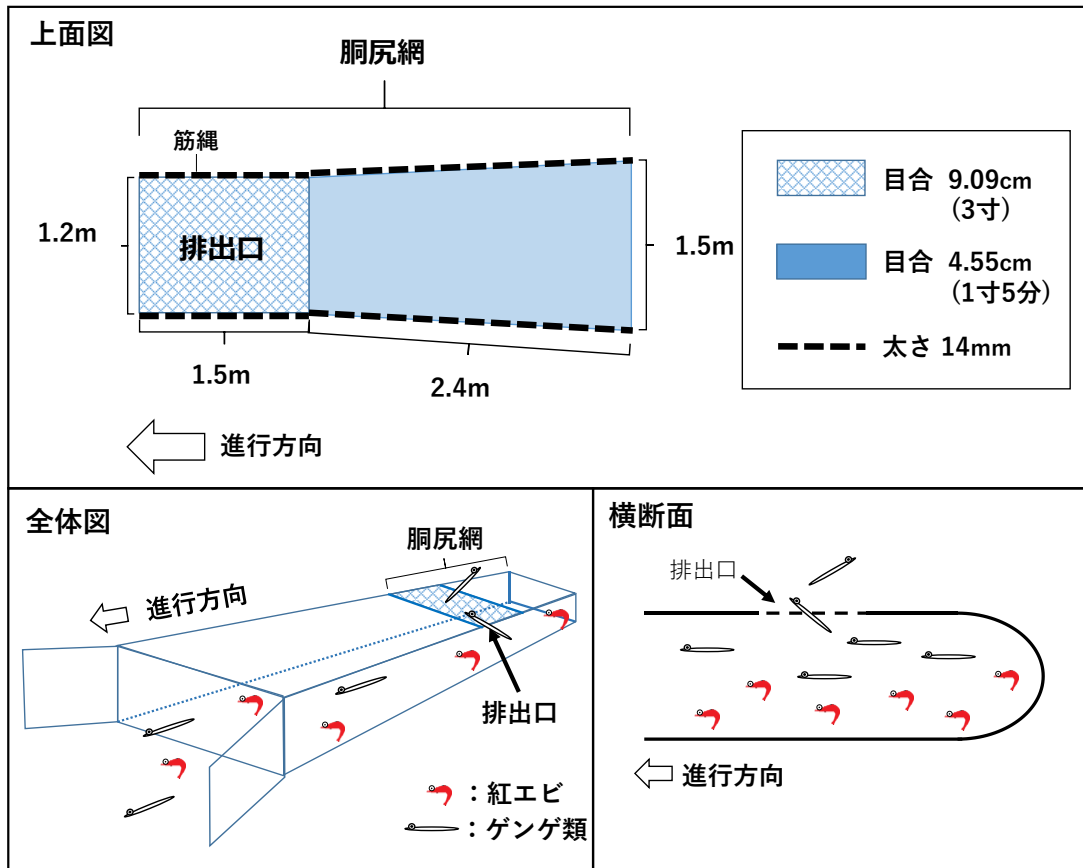
図1 胴尻網の改良部
