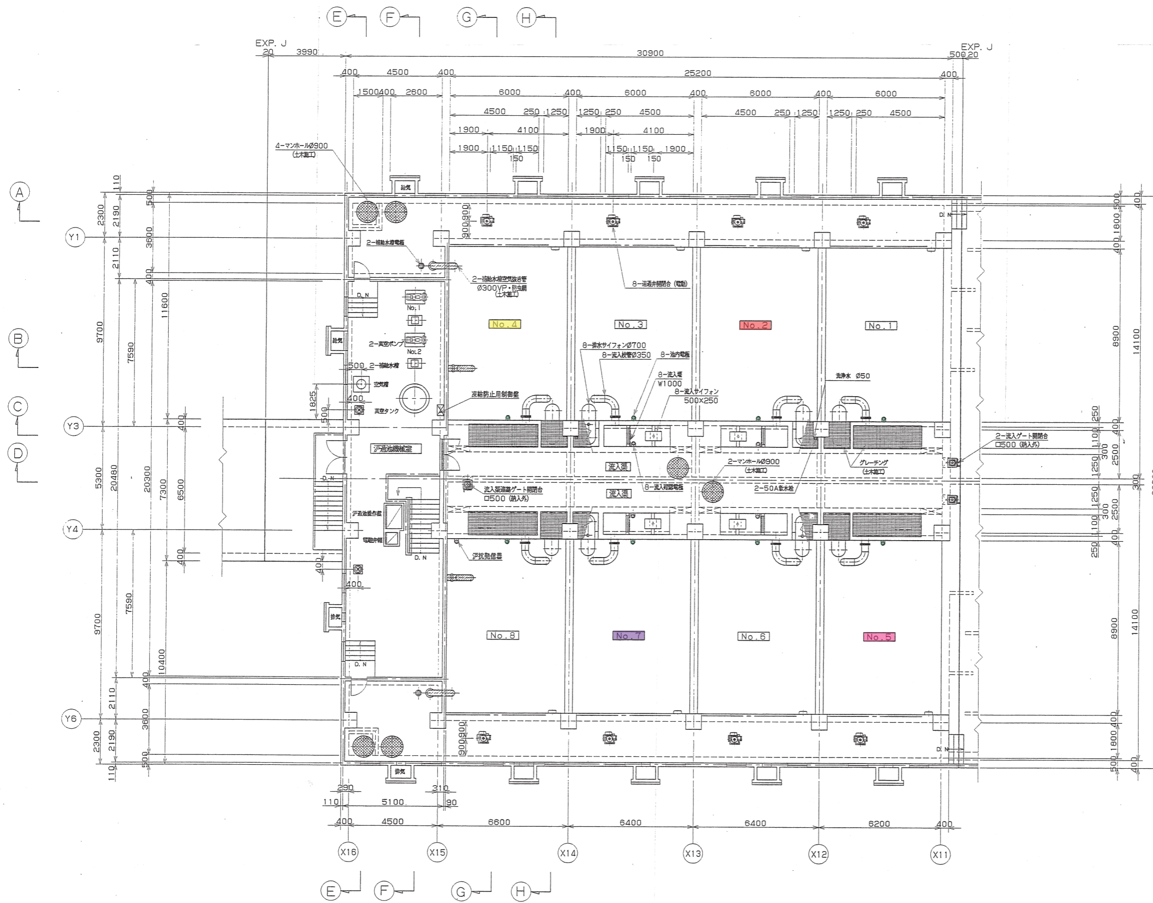
平面図(その1) S=1/200
