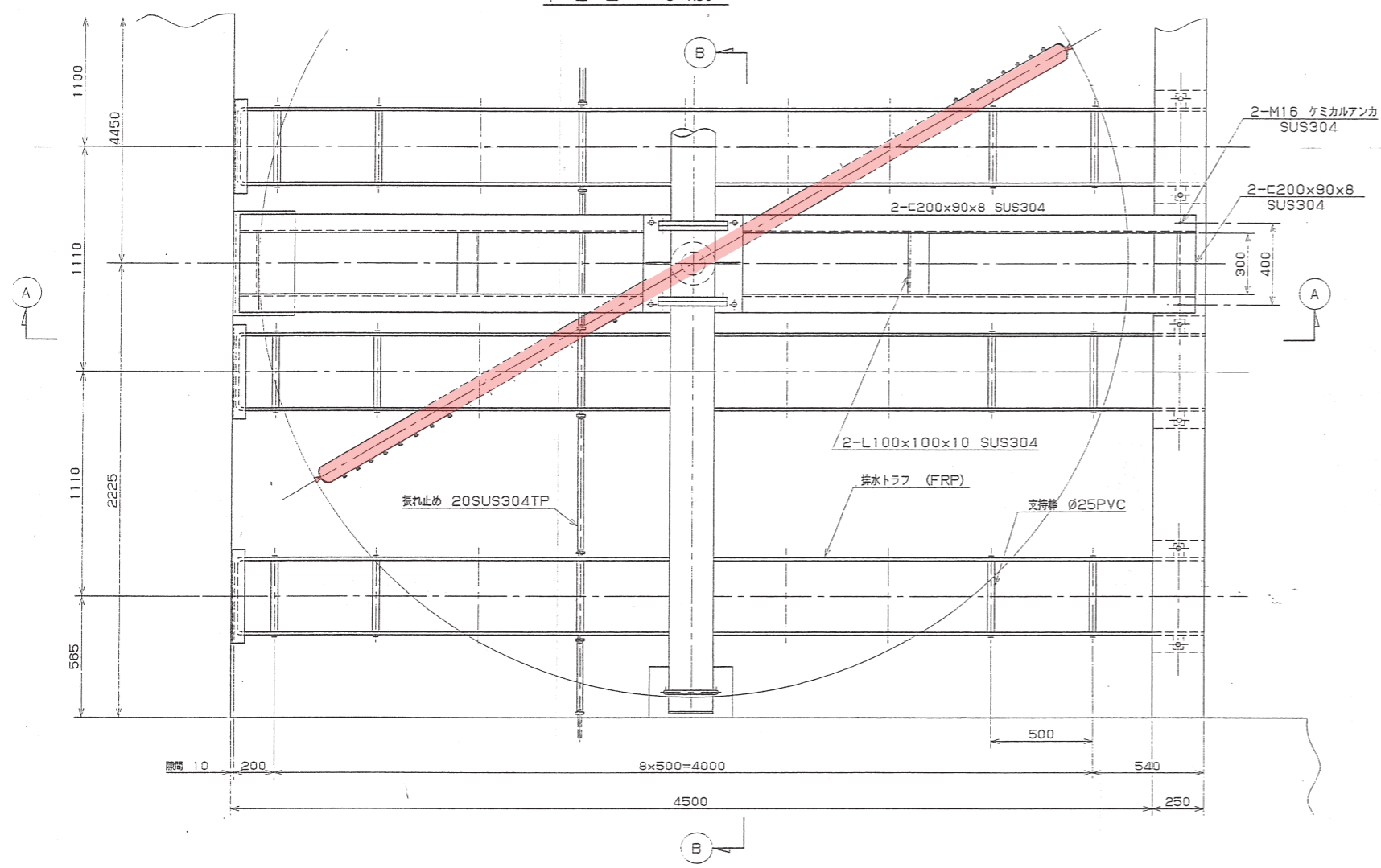
平面図 S=1:30
