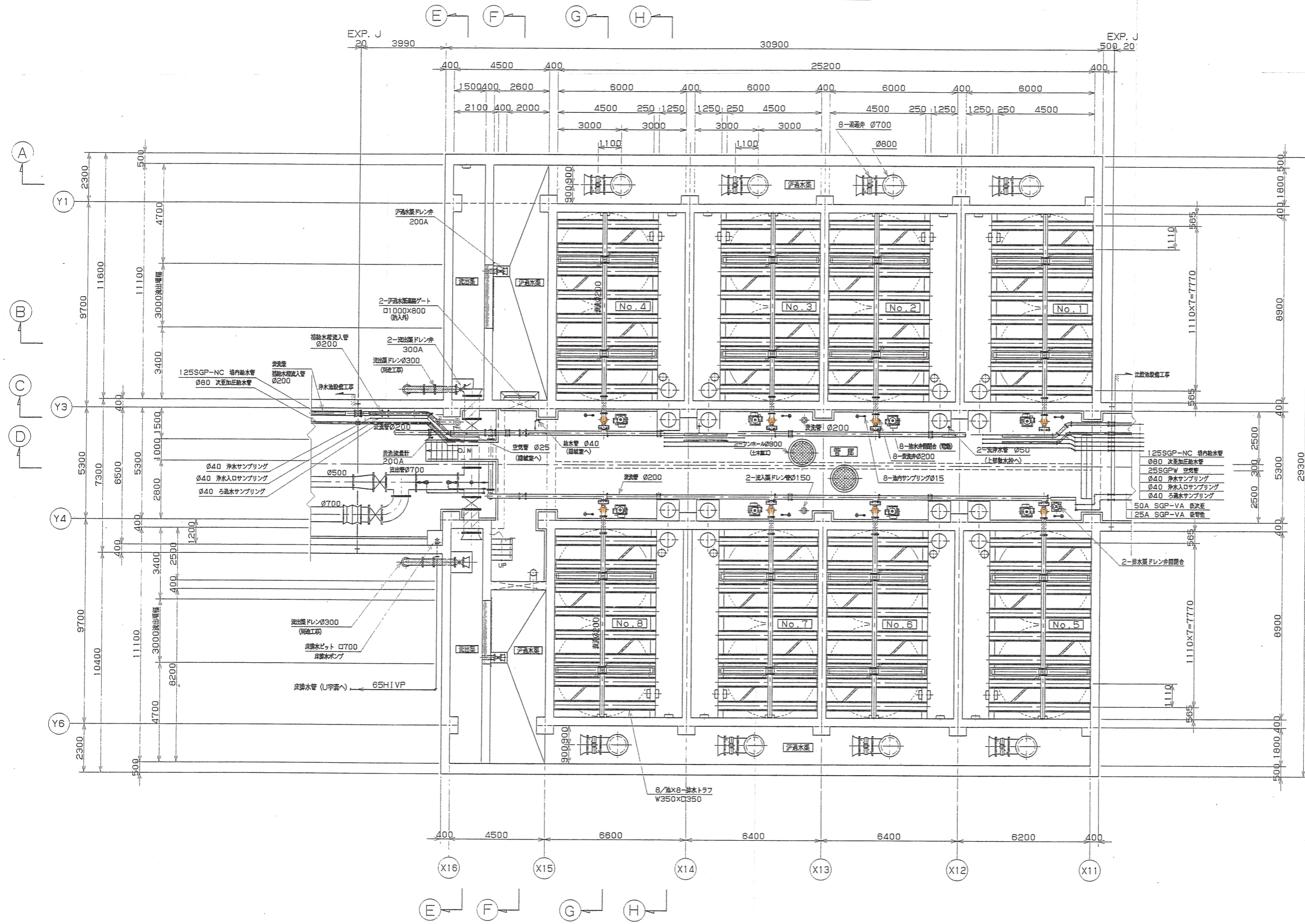
平面図(その3) S=1/200
