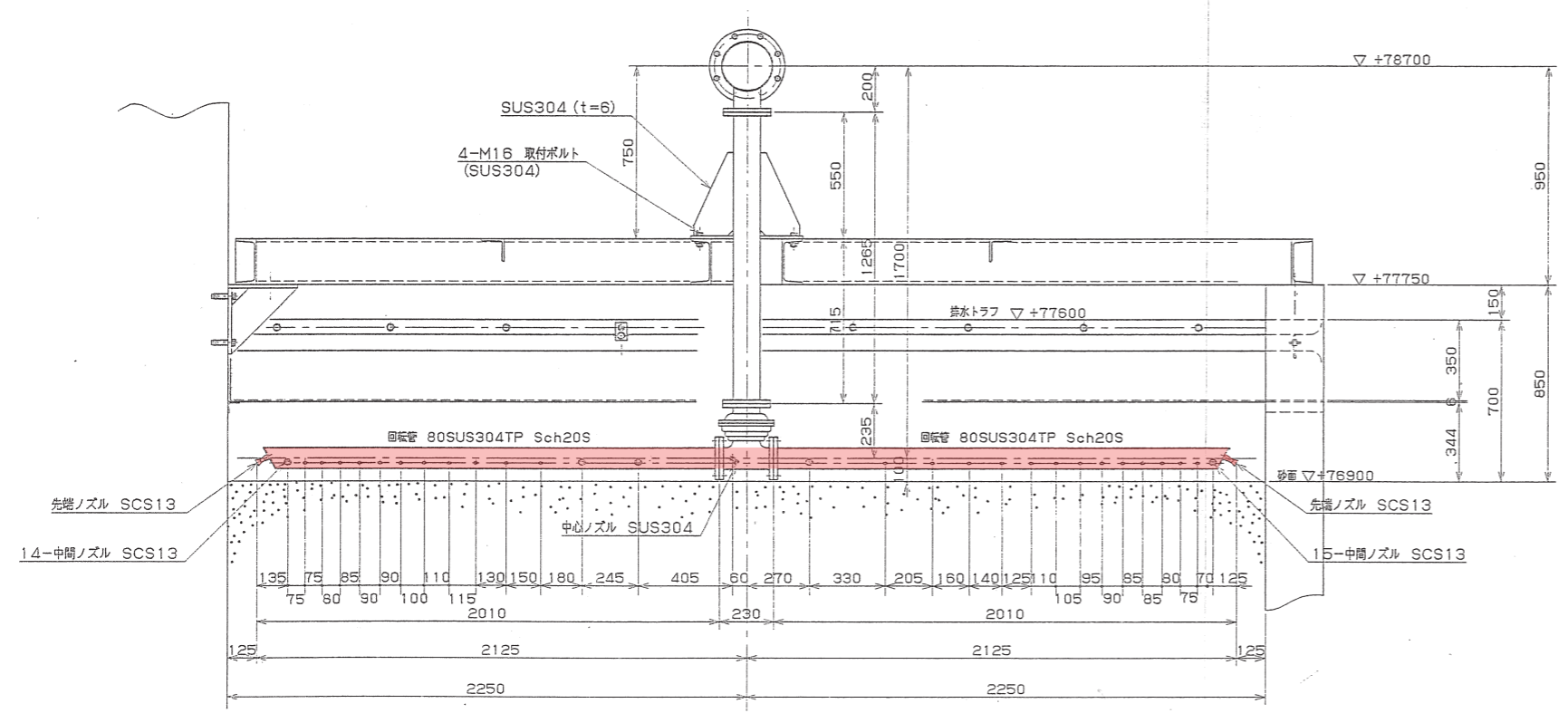
断面図 S=1:30
