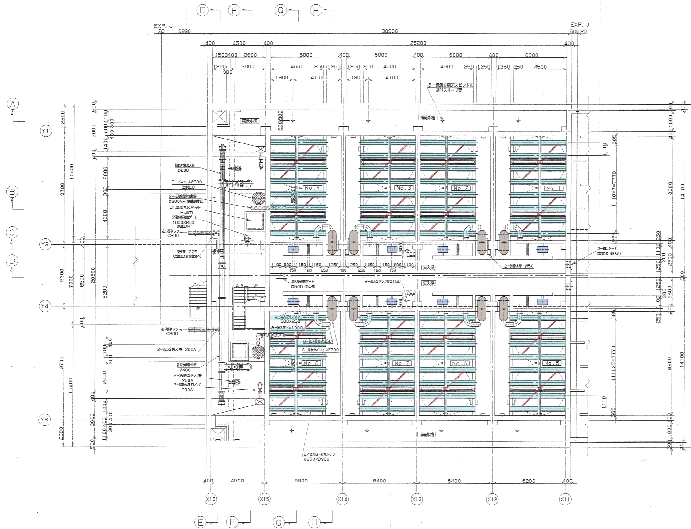
平面図(その2) S=1/200
